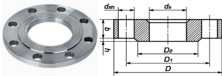
Фланец ГОСТ Ру10
