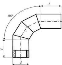
відвід 90° двосекційний
