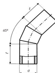
відвід 45° односекційний
