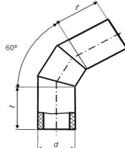
відвід 60° односекційний
