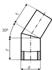
відвід 30° одностикової
