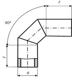
відвід 90° односекційний
