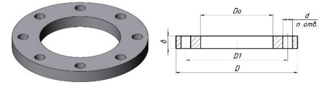
Фланец Покр Ру10
