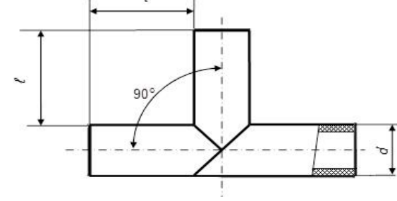
Трійник
