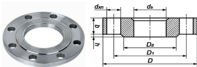
Фланец ГОСТ Ру10
