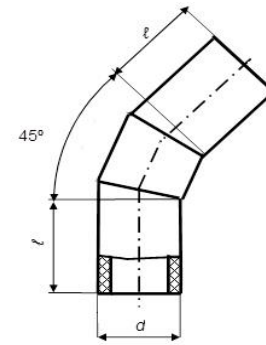
відвід 45° одностикової
