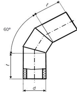
відвід 60° односекційний
