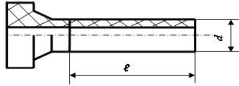
Втулка подовжена
