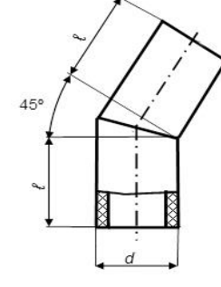
відвід 45° одностикової
