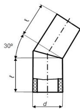
відвід 30° одностикової
