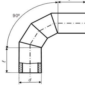
відвід 90° двосекційний
